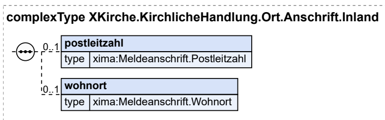
Abbildung II.3.7. XKirche.KirchlicheHandlung.Ort.Anschrift.Inland
