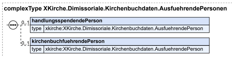
Abbildung V.5.12. XKirche.Dimissoriale.Kirchenbuchdaten.AusfuehrendePersonen
