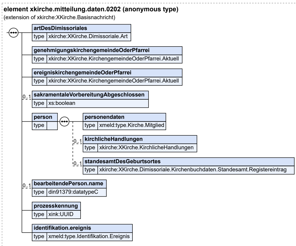
Abbildung V.6.2. xkirche.mitteilung.daten.0202
