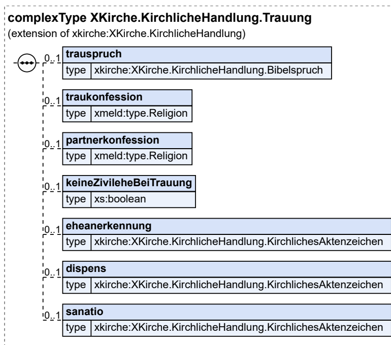
Abbildung II.3.15. XKirche.KirchlicheHandlung.Trauung
