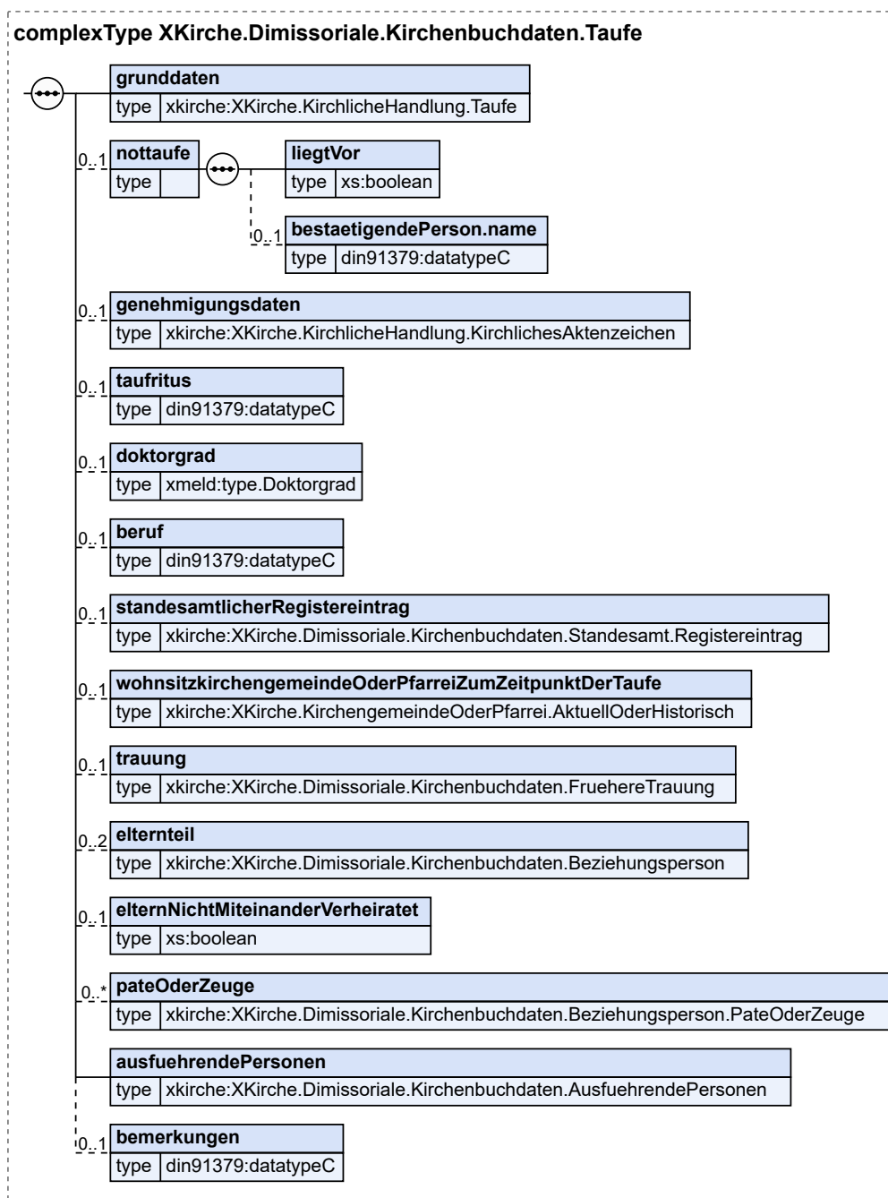
Abbildung V.5.8. XKirche.Dimissoriale.Kirchenbuchdaten.Taufe
