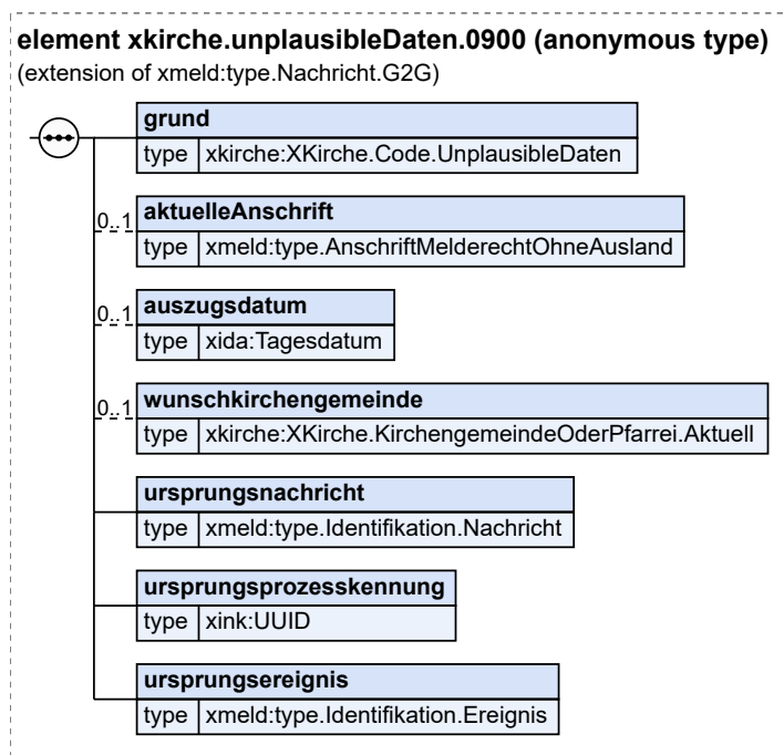
Abbildung V.6.5. xkirche.unplausibleDaten.0900
