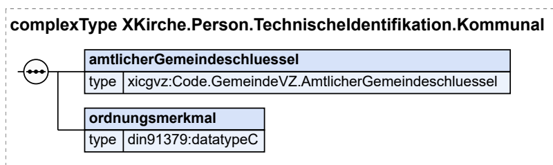
Abbildung II.3.28. XKirche.Person.Technischeldentifikation.Kommunal
